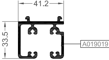
Ölçek / Scale 1:2
