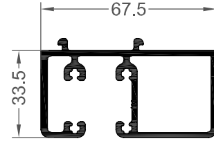
Ölçek / Scale 1:2
