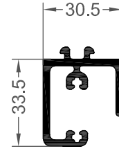
Ölçek / Scale 1:2
