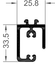
Ölçek / Scale 1:2
