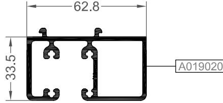
Ölçek / Scale 1:2
